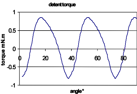
Fig 5: Detent torque.
