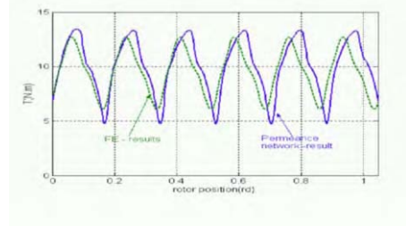
Fig. 5. Dynamic torque
