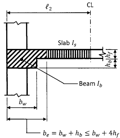
Edge beam
