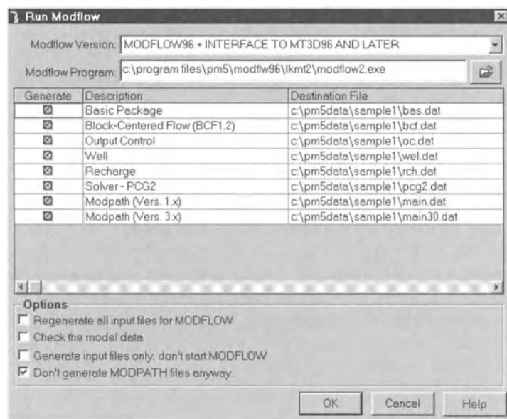
Fig. 2.7. The Run Modflow dialog box
