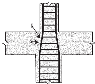
Fig. 10.4.2.10—Longitudinal bar offset.
