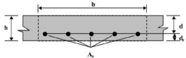
Fig. 7.3.4.2—Slab section.
