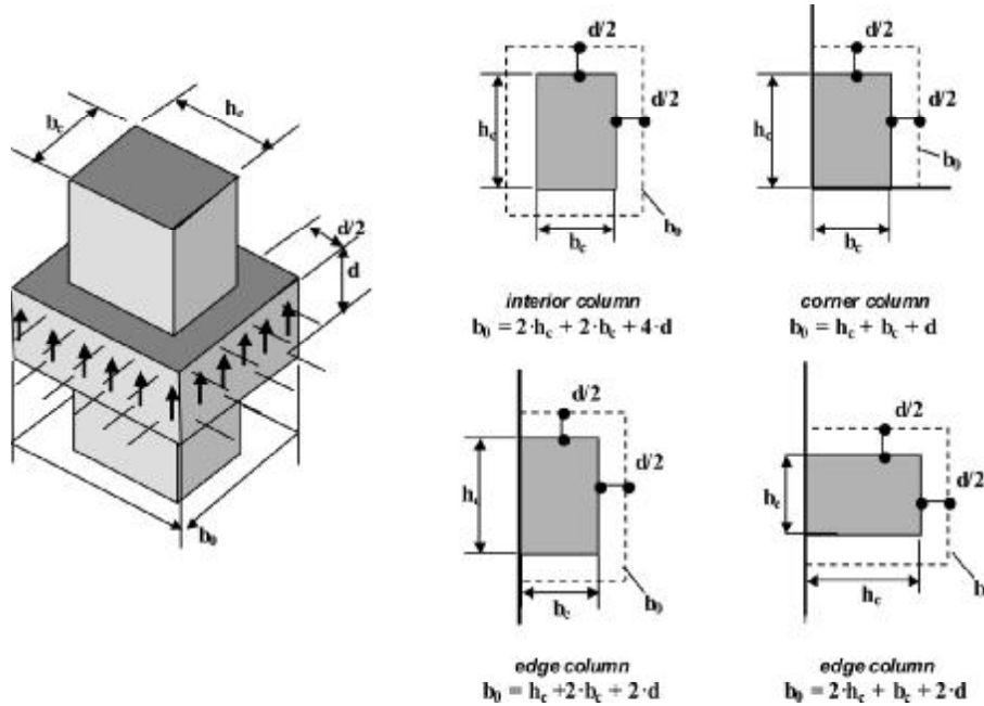
Fig. 9.5.4.2—Definition of b_o .
