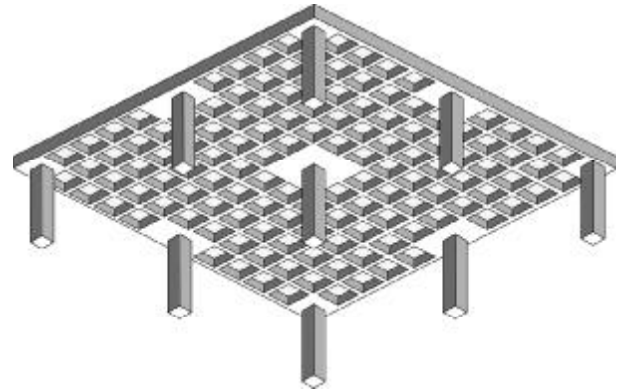
Fig. 6.1.4.4—Waffle-slab.
