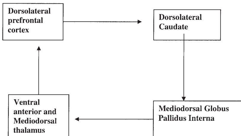
Fig. 4. Dorsolateral circuit.
