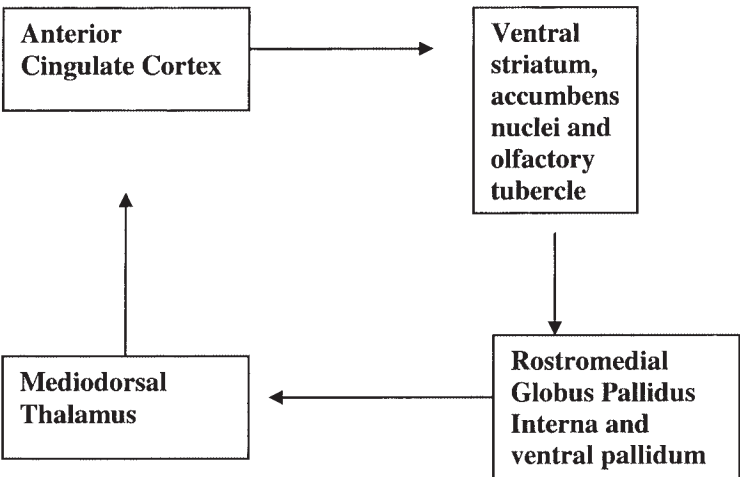
Fig. 2. Cingulate circuit.
