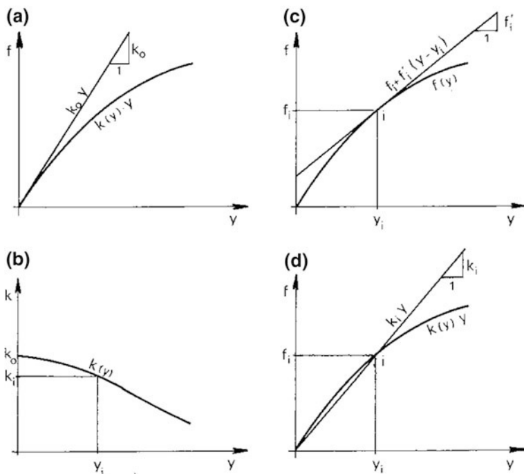
Fig. 6.35 Initial (a), variable (b), tangent (c) and secant (d) stiffness
